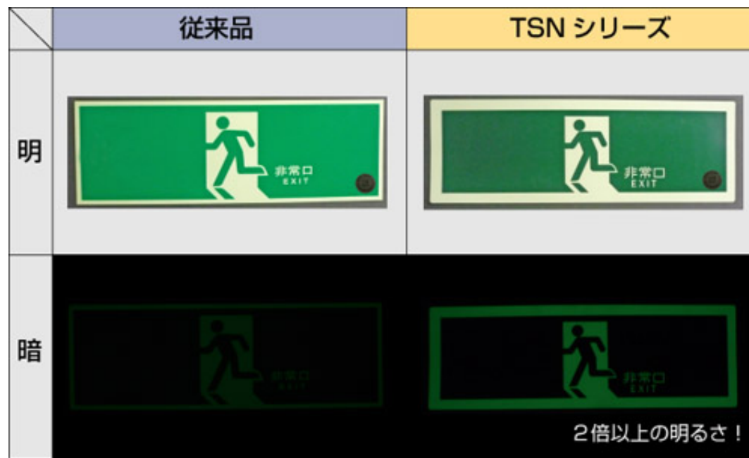
従来品(硬質樹脂プレート)との輝度比較
