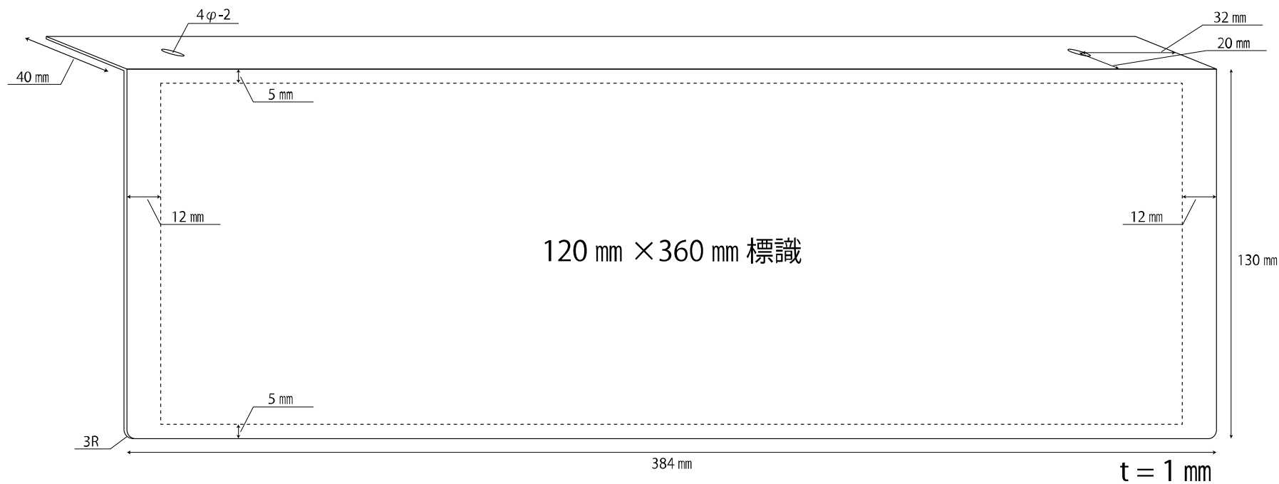
天井用塩ビプレート (白色)
