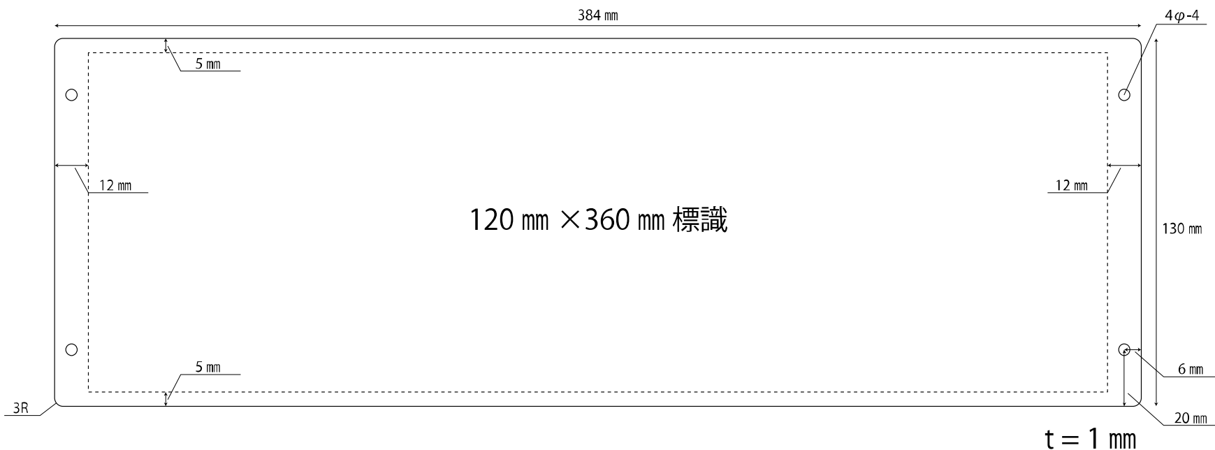
壁面用塩ビプレート (透明)
